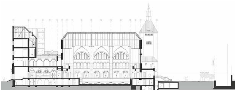
Längsschnitt • Longitudinal section
